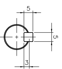
<축단 치수 상세도>
