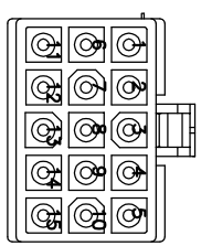
Plug 사양:172171-1 (AMP)
